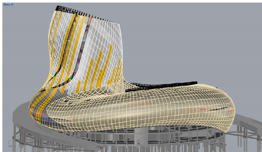
Modélisation complète de la structure du lot 01 : béton, charpente bois, vêtire métal et vêtire verre
