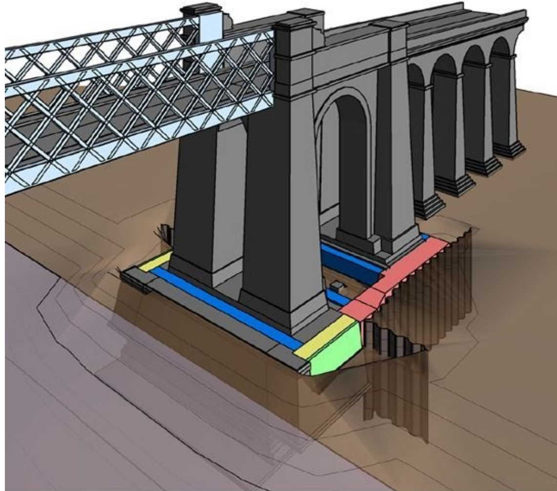
Stabilisation pile-culée
