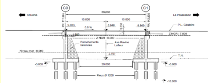
COUPE LONGITUDINALE BRETELLE 2
