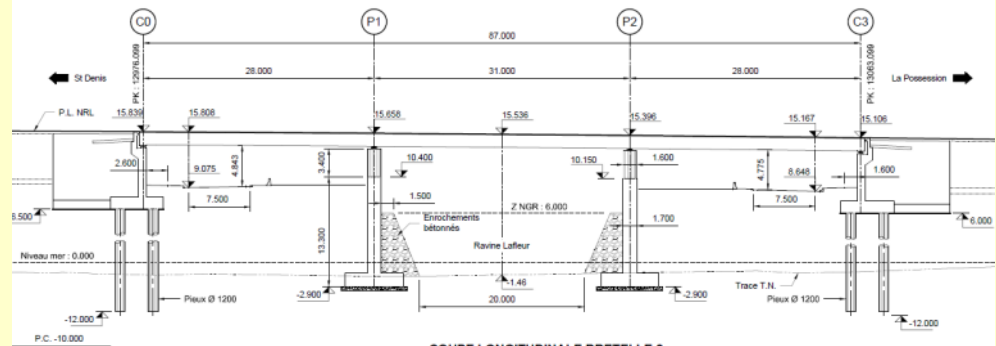
COUPE LONGITUDINALE BRETELLE 2
