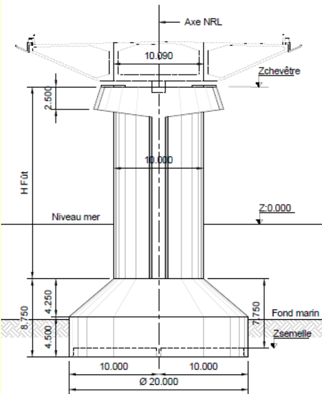
ÉLÉVATION TRANSVERSALE
