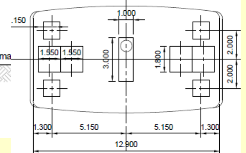
DÉTAIL CHEVÊTRE
